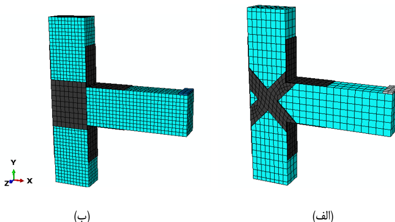
شکل ۳- مش بندی مدل اتصال تیر-ستون تقویت شده با CFRP در چیدمان: (الف) نخست و (ب) دوم (خروجی نرم افزار ABAQUS، مدل سازی حاضر)
