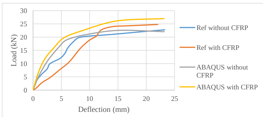
شکل ۴- مقایسه نمودار نیرو - جابه‌جایی نتایج مدل‌سازی با داده‌های مرجع برای حالت‌های تقویت‌نشده و تقویت‌شده با CFRP [تحلیل حاضر مبتنی بر داده‌های ۲]
